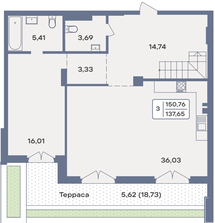
1 ЭТАЖ
